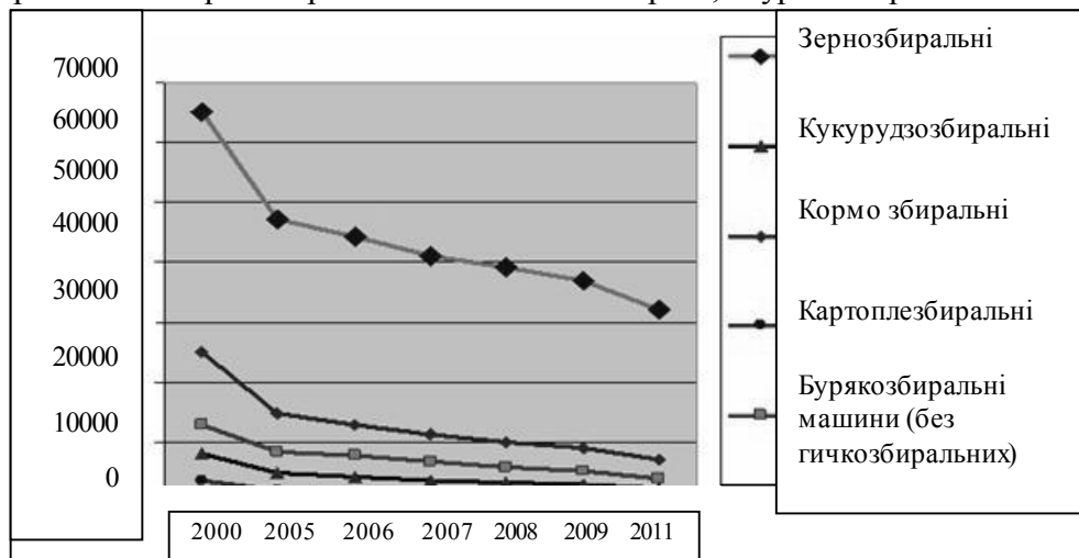
Рис. 1. Структура сільськогосподарської техніки по роках її випуску в господарствах України
